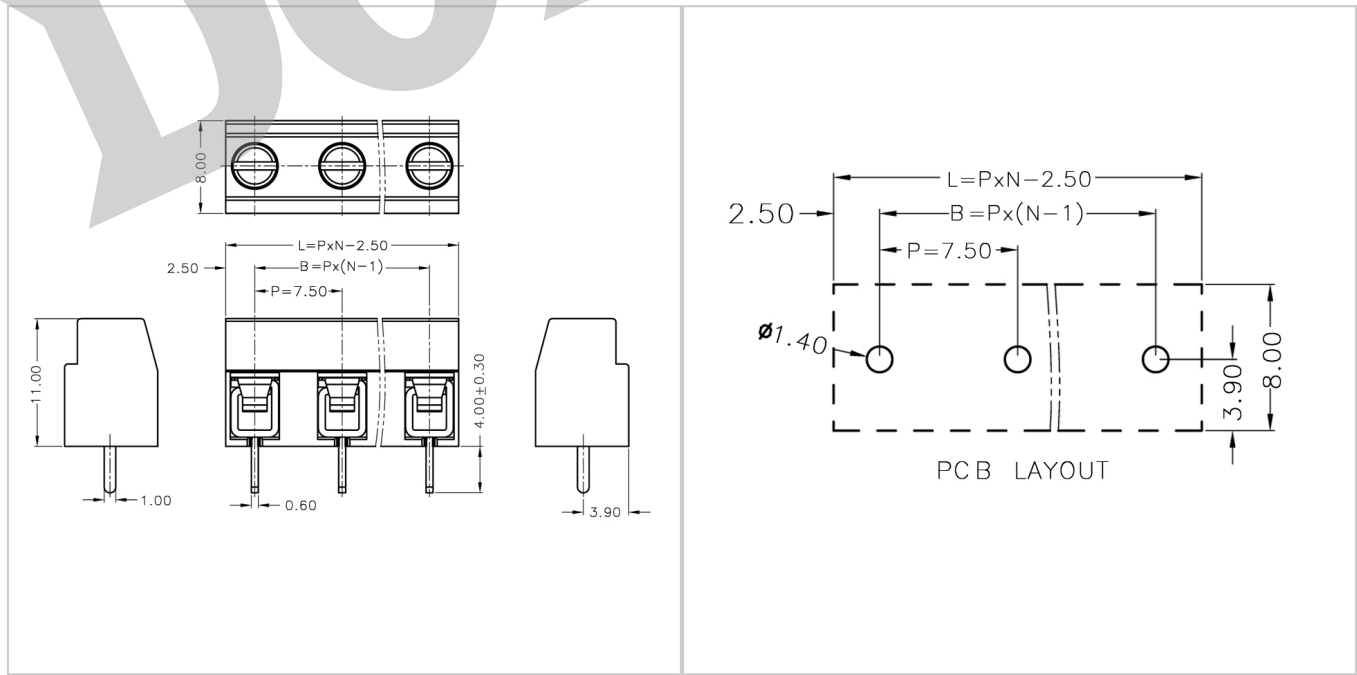
尺寸图
