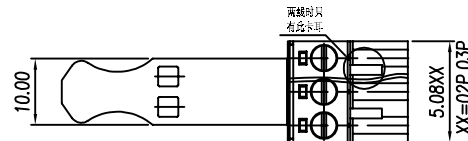
02~03P尺寸图
