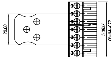
04~07P尺寸图
