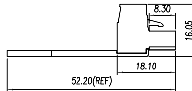
04~07P尺寸图
